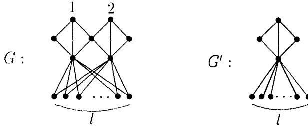
Fig. 1. d_v(G) < d_v(G') .
